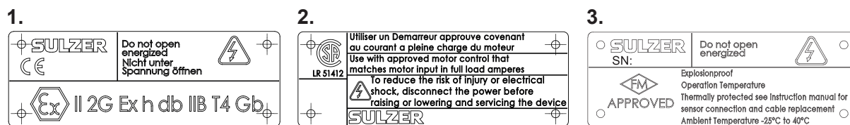
Slika 5. Napisne ploščice Ex
