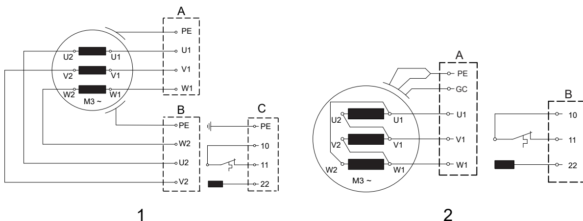
Slika 14. (1) 50 Hz: Dva napajalna kabela in en krmilni kabel. (2) 60 Hz: En napajalni in en krmilni kabel.
