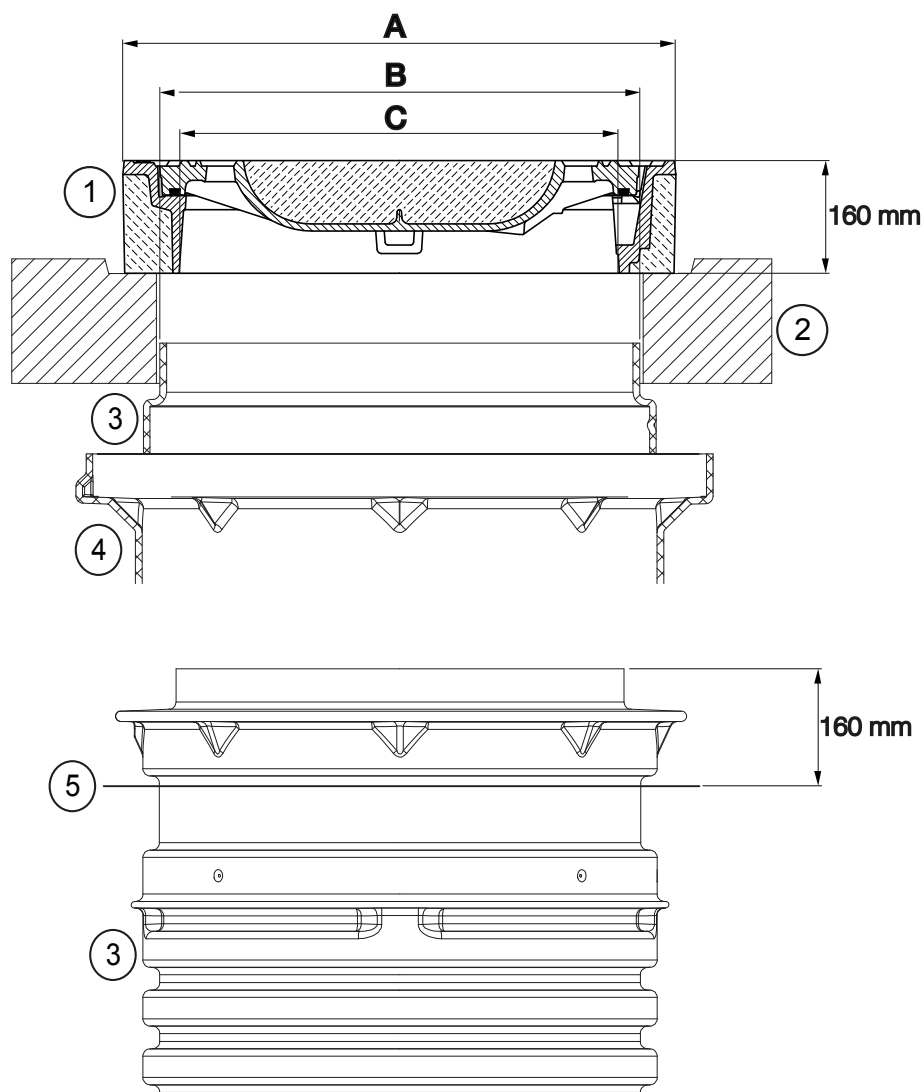
Bild 16. Lock av klass D400 – tvärsnittsrörning och mått
