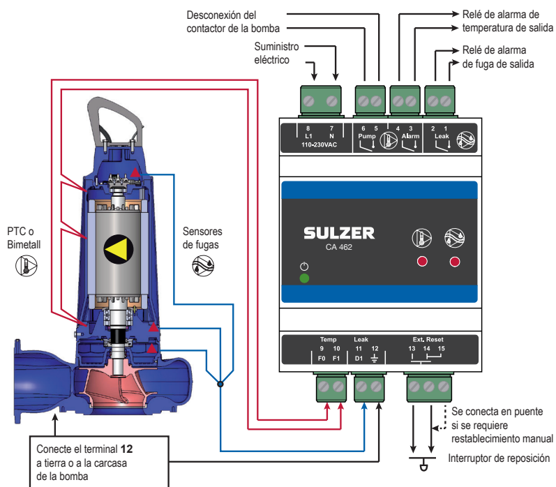
Figura 1 Diagrama de conexiones eléctricas
