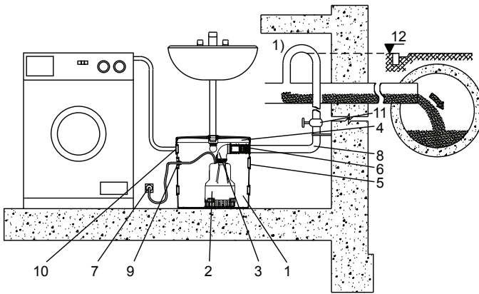
Kuva 5: Asennusesimerkki
