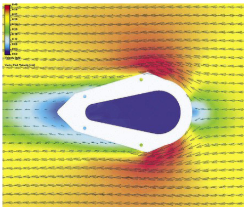
CFD Analyse zum Betonsockel
