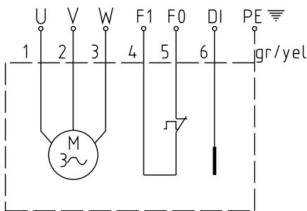
Figura 6: Esquema de conexiones trifásicas con limitador de temperatura y DI
