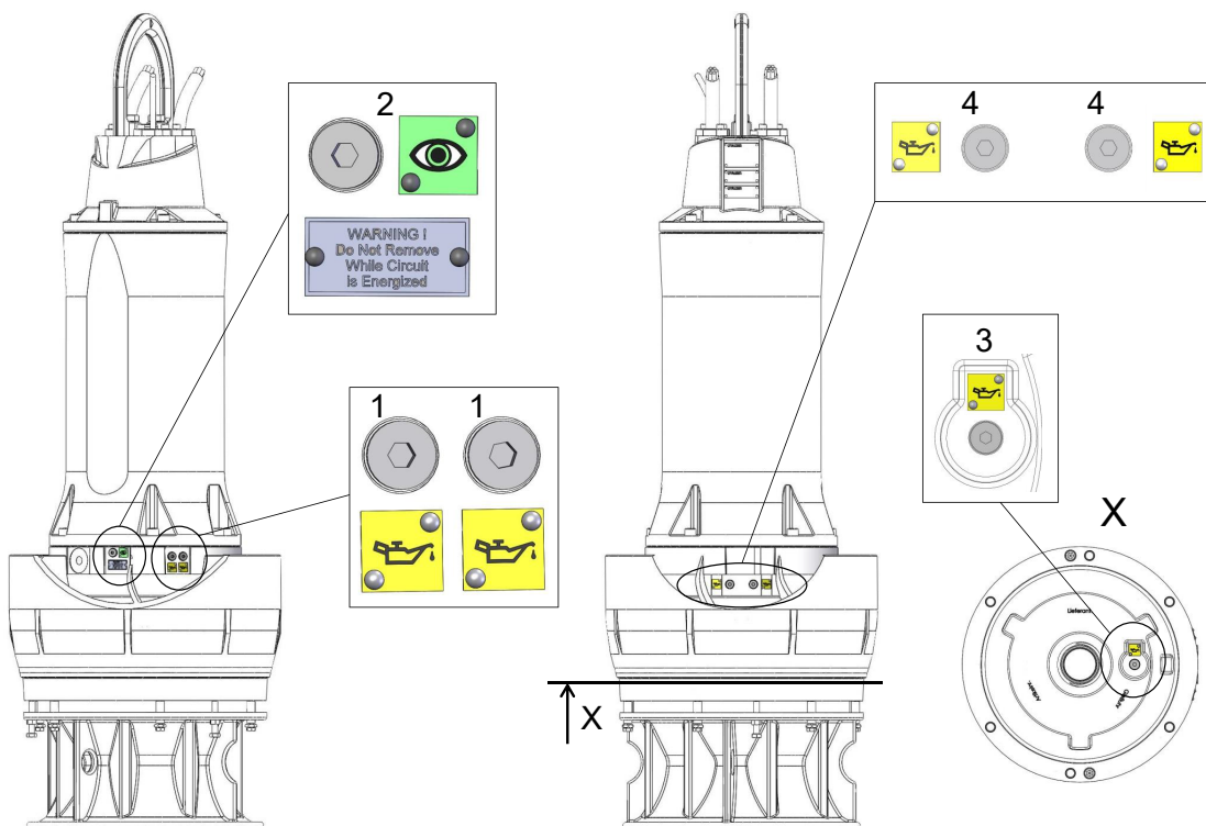
Illustration 24. Oljepåfyllning och -tömning AFLX / VUPX PE4
