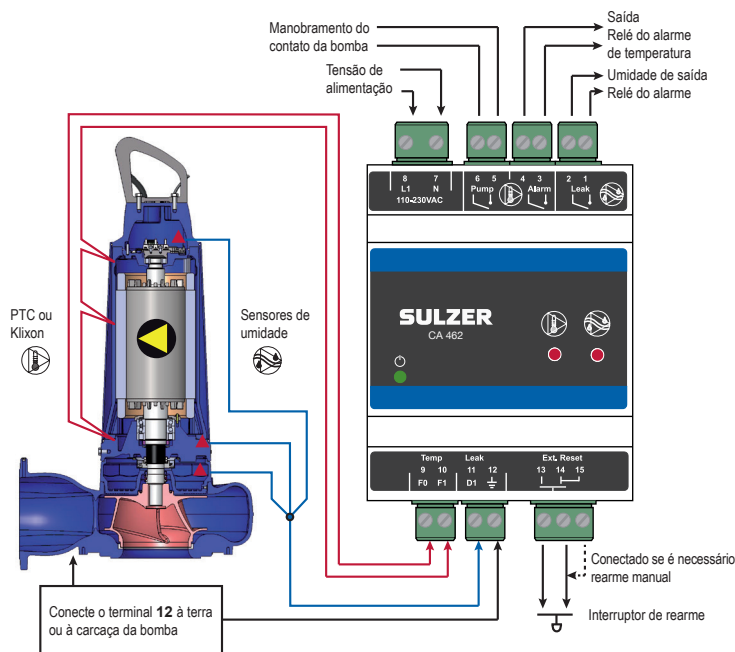
Figura 1 Diagrama de conexões elétricas
