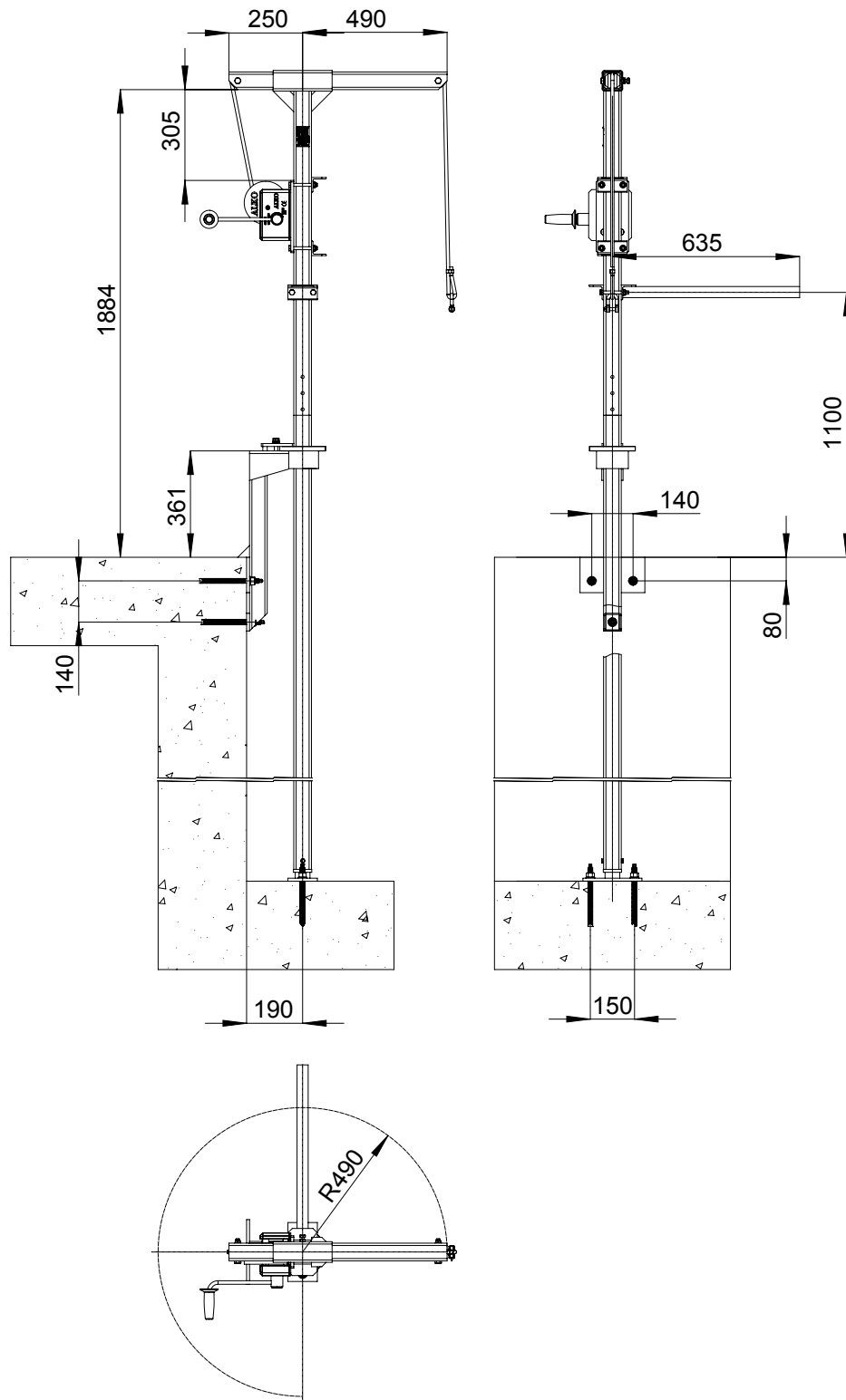
Εικ. 1 Διαστάσεις κατασκευής
