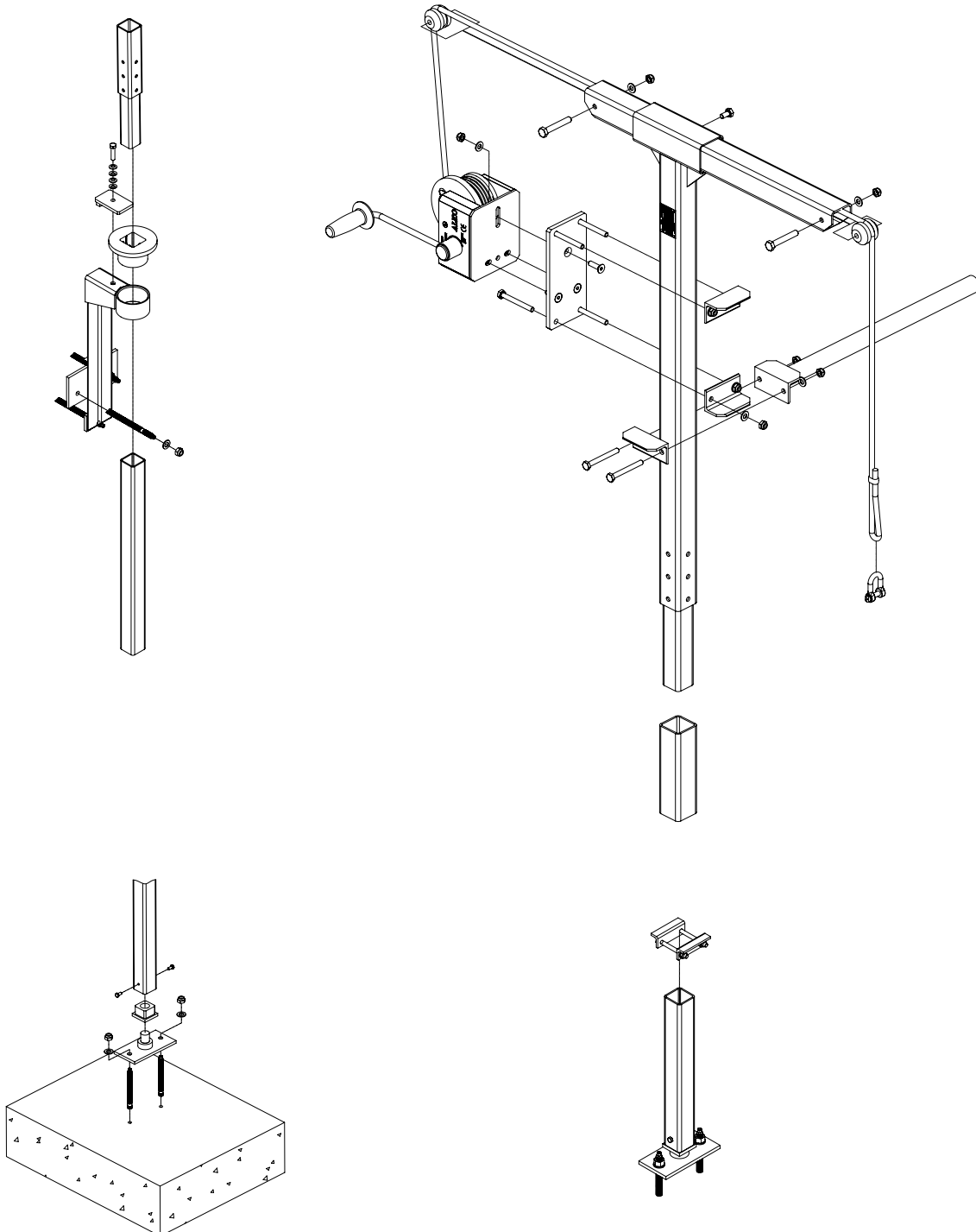
Εικ. 4 Τοποθέτηση/αφαίρεση της συσκευής ανύψωσης
