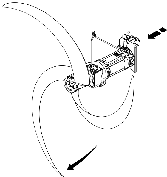
Obr. 22 Kontrola směru otáčení XSB 2750
