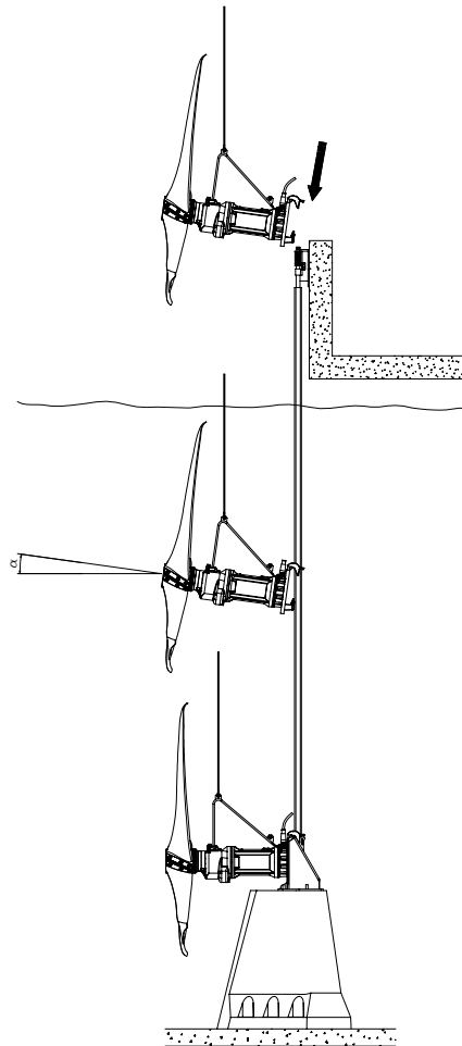
Obr. 25 Spuštění akceleračního proudění
