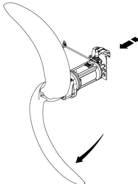
Obr. 23 Kontrola směru otáčení XSB 2500
