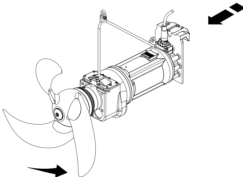
Obr. 24 Kontrola směru otáčení XSB 900
