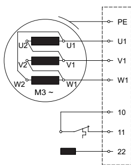
Obr. 17 Kabel pro připojení motoru s integrovanými řídicími vodiči
