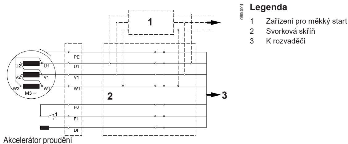
Obr. 20 Návrh zapojení motoru se zařízením pro měkký start (volitelné příslušenství)
