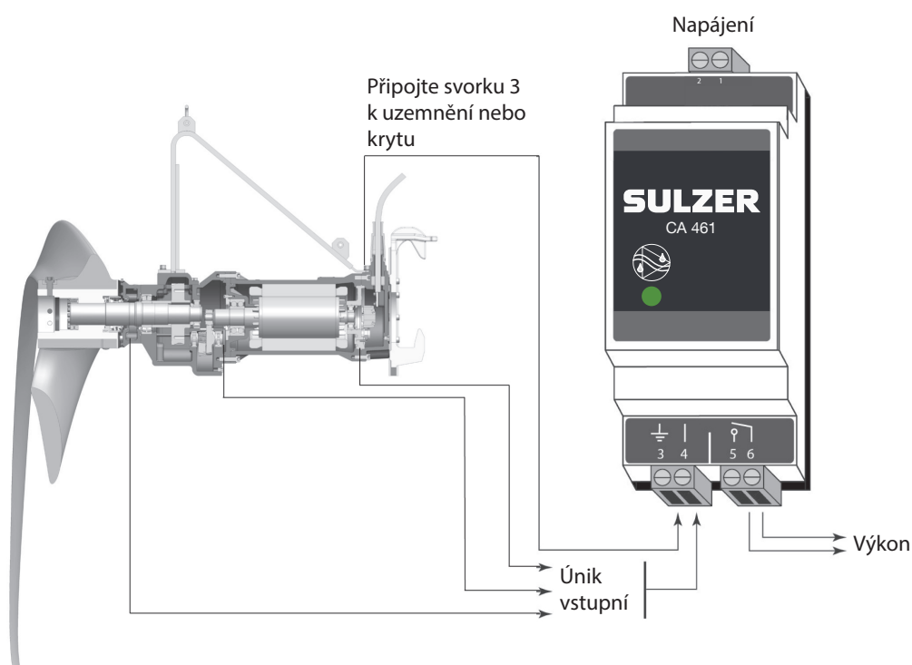
obr. 25 Zesilovač se světelným signalizačním zařízením
