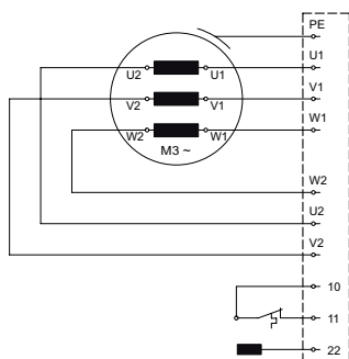
Obr. 18 Kabel pro připojení motoru s integrovanými řídicími vodiči
