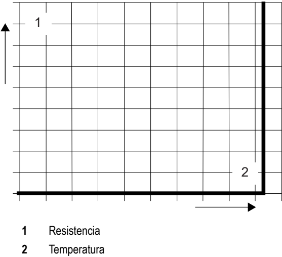
Figura 11. Curva que muestra el principio de funcionamiento del limitador de temperatura bimetalico
