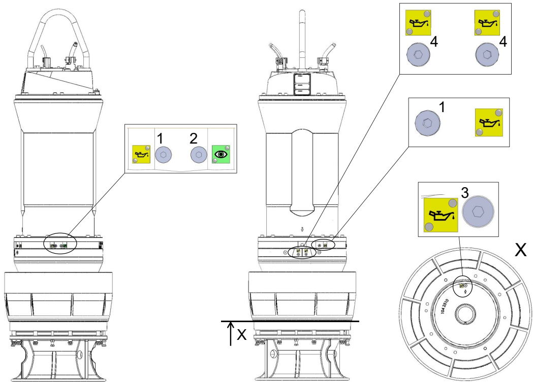
Figura 26. Llenado y vaciado de aceite AFLX / VUPX PE6
