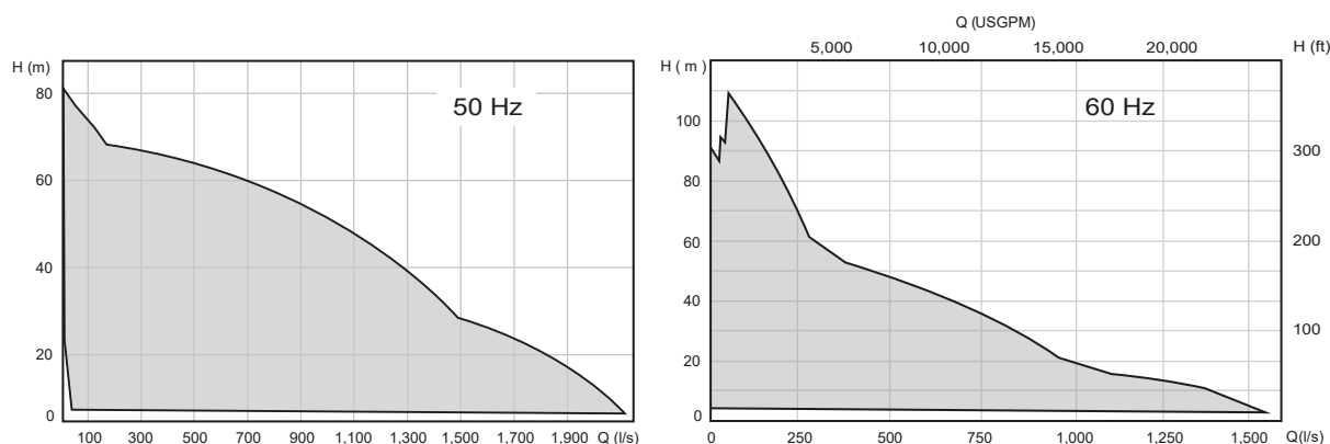
Figura 1. XFP 50 Hz / 60 Hz
