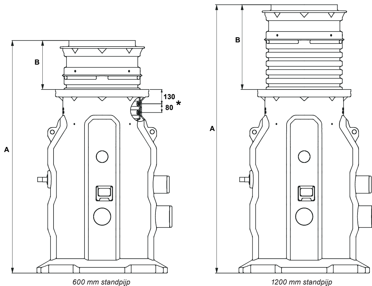
Figuur 6. Tank- en standpijpmetingen
