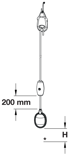
Figuur 10. Instelling vlotterschakelaar
