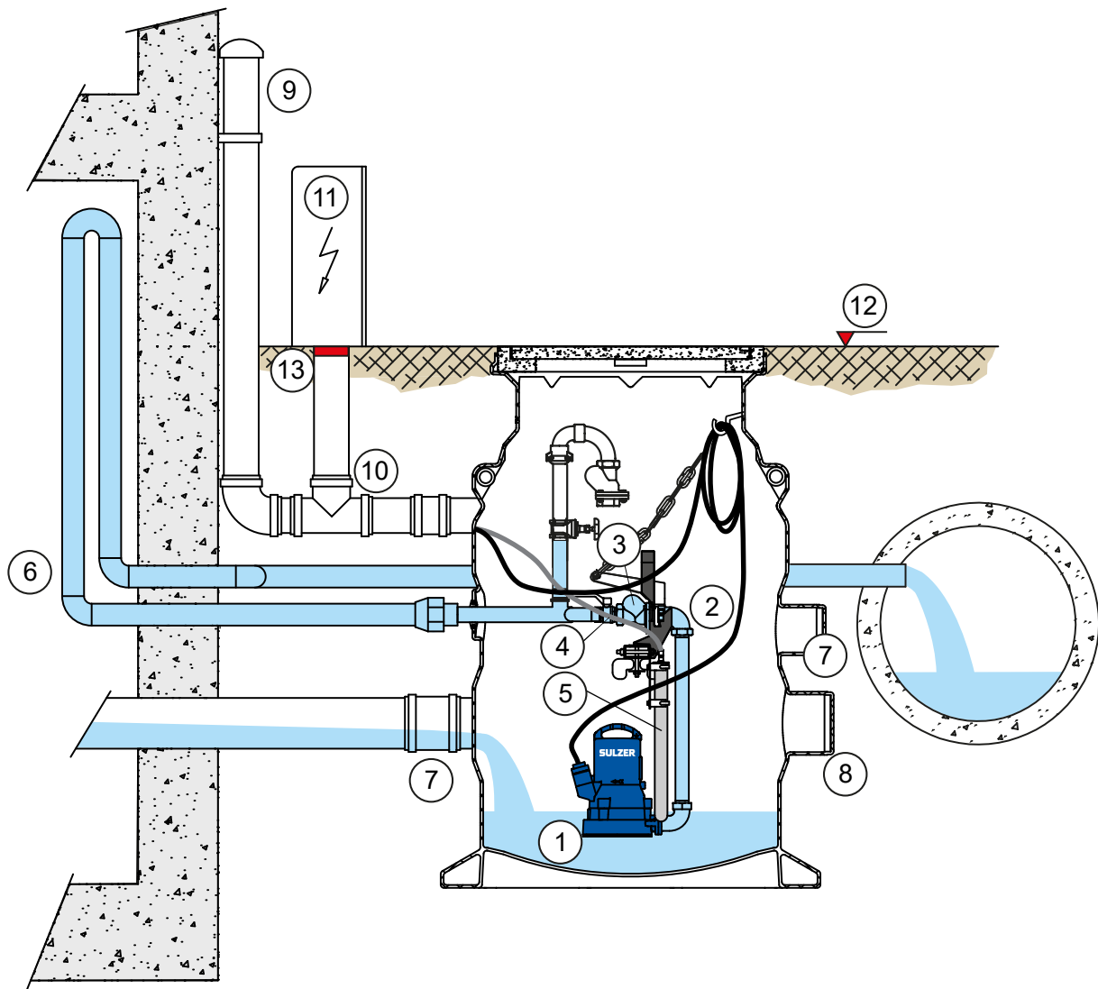
Figuur 1. Installatievoorbeeld
