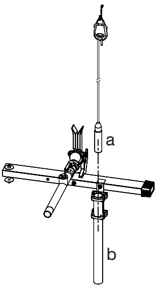
Figuur 9. Vlottersensor
