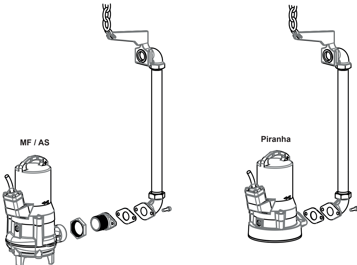
Figuur 2. Pompuittloopaansluitingen
