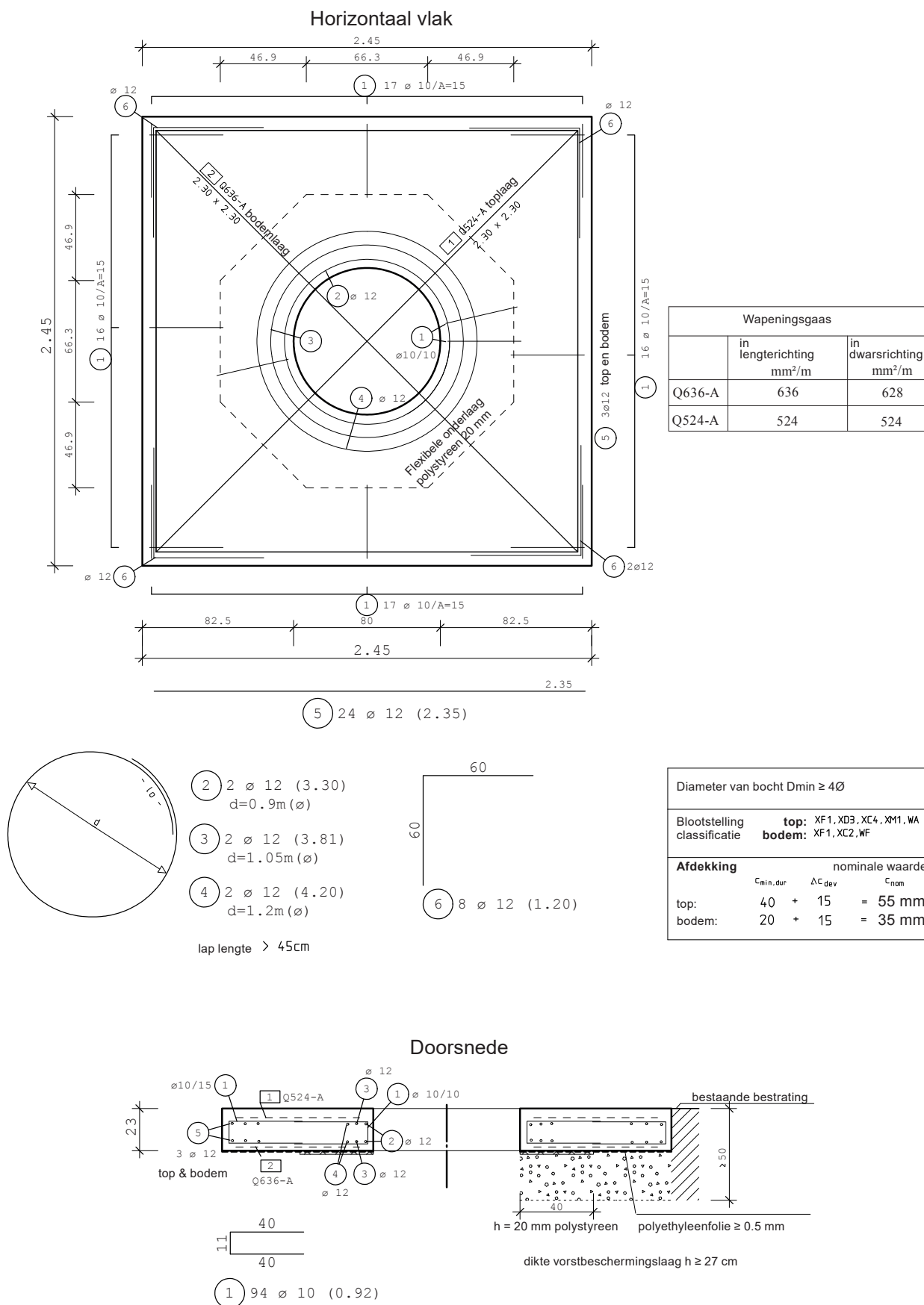
Figuur 5. Specificatie en afmetingen verdeelplaat
