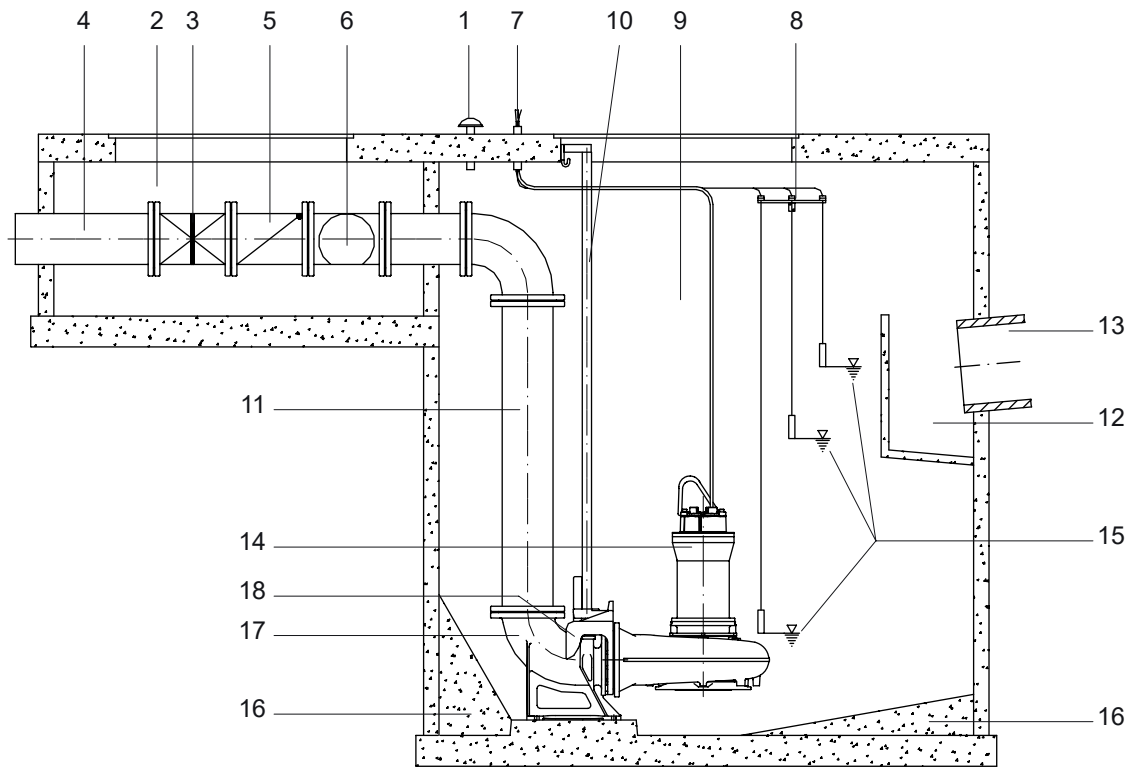
Figure 5. Installation humide (verticale) avec système d'accouplement automatique Sulzer
