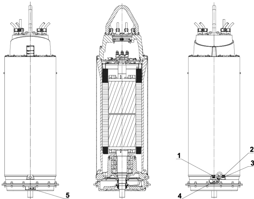
Figure 17. Remplissage et vidange d'huile XFP PE7
