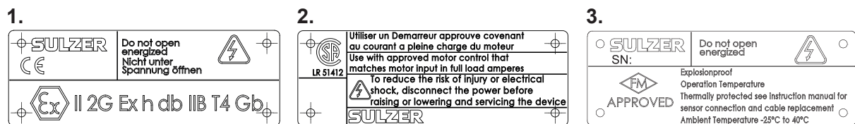
Figure 2. Plaques signalétiques Ex
