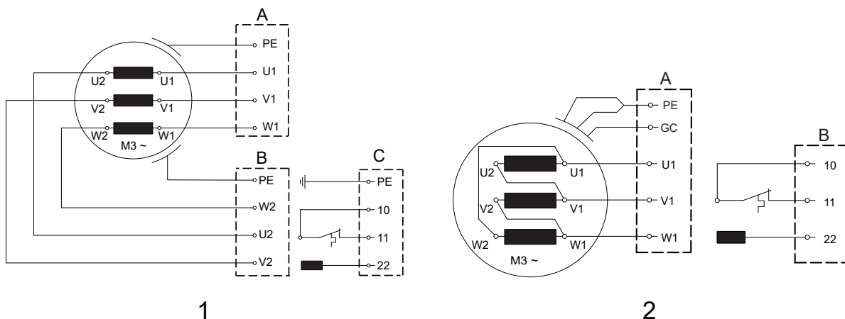
Figure 14. (3) Versions spéciales 50 Hz : Deux câbles d'alimentation et un câble de commande - pour fonctions de surveillance du moteur en option.
