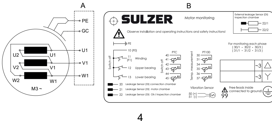
Figure 15. (4) 60 Hz: Un câble d'alimentation et un câble de commande - pour fonctions de surveillance du moteur en option.
