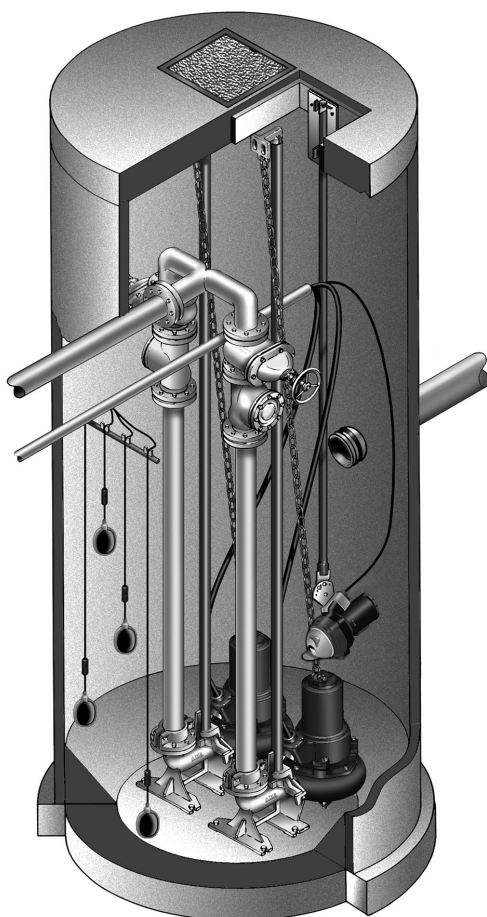
Geleidebuis
