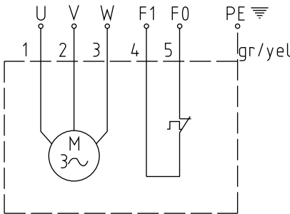
Figure 6: Câblage triphasé avec limiteur de température
