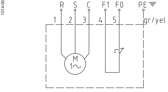
Figure 9: Câblage monophasé avec limiteur de température
