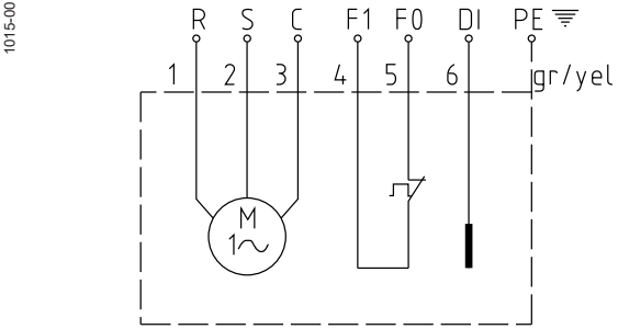
Figure 10: Câblage monophasé avec limiteur de température et DI
