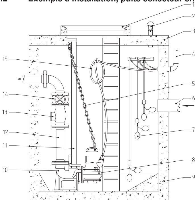
Figure 3 Exemple d'installation, puits collecteur en béton
