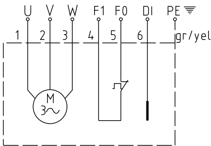
Figure 7: Câblage triphasé avec limiteur de température et DI
