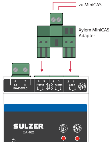
Abbildung 3 Anschlussdiagramm MiniCAS Adapter
