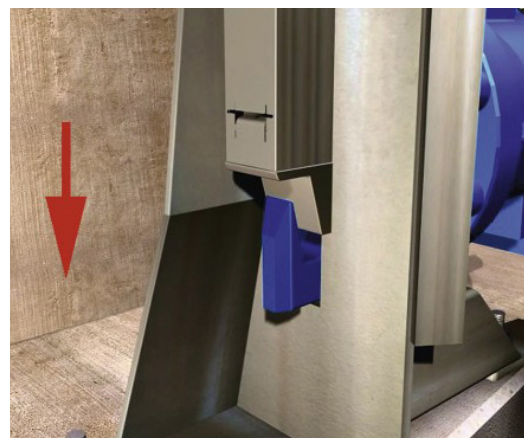
定位 (内视图)
