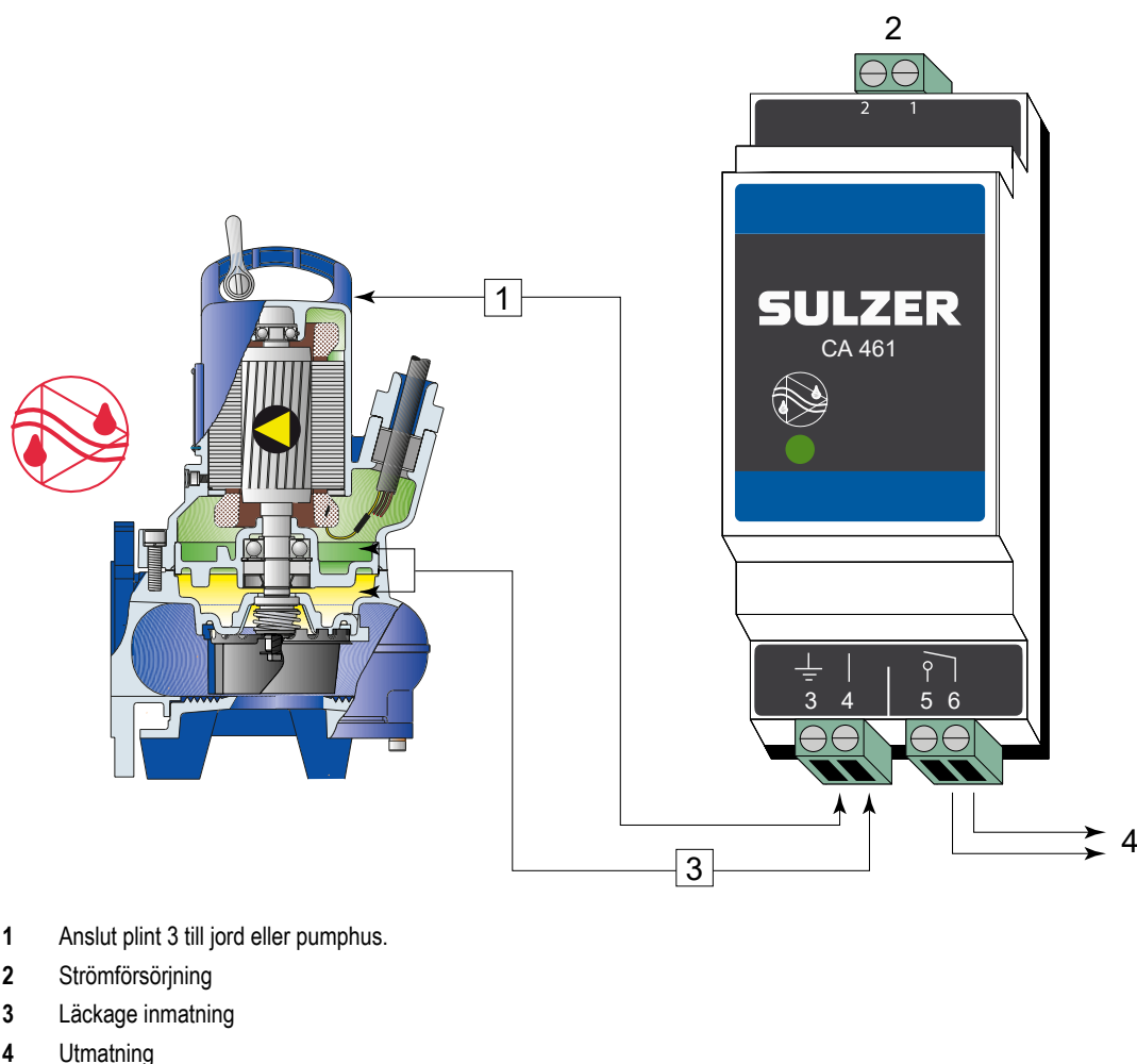
Illustration 5. Sulzer läckagekontroll typ CA 461
