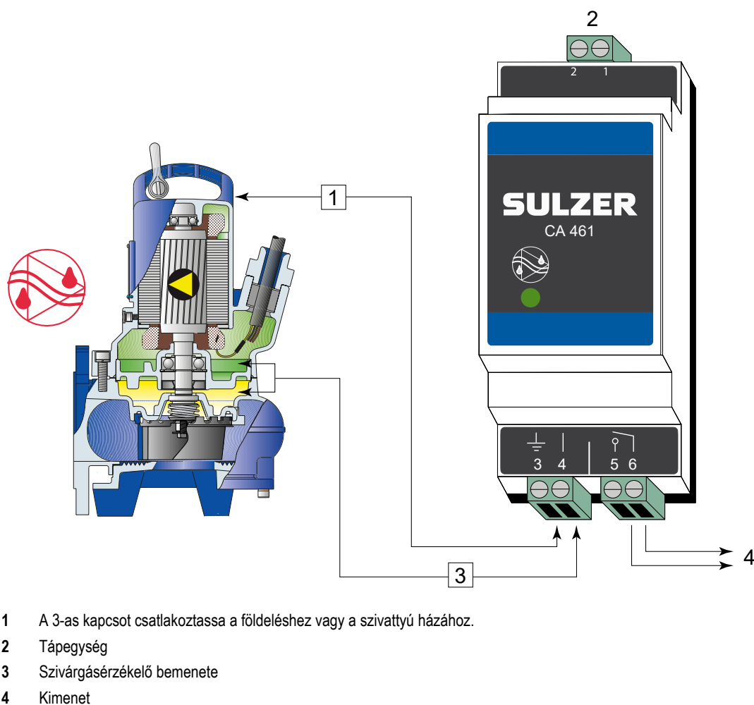
Ábra 5. Sulzer CA 461 típusú szivárgásellenőrző
