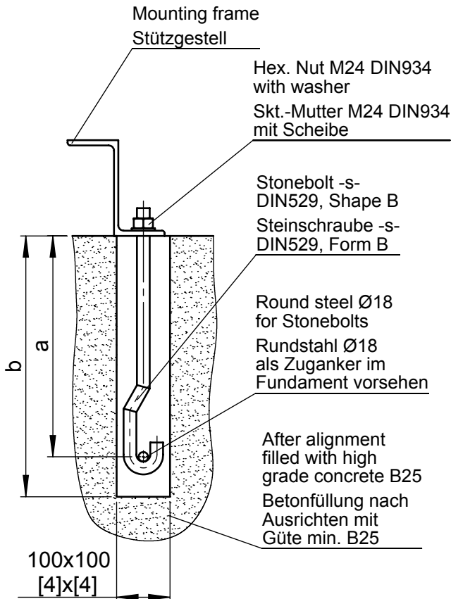
View of stonebolt anchorage Ansicht Steinschraubenverankerung
