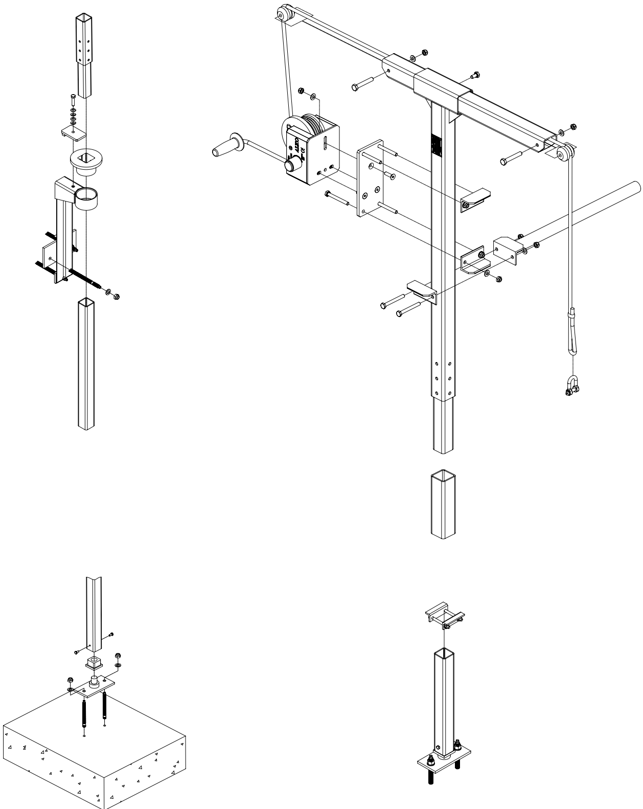
Figura 4 Montagem/desmontagem do aparelho de elevação
