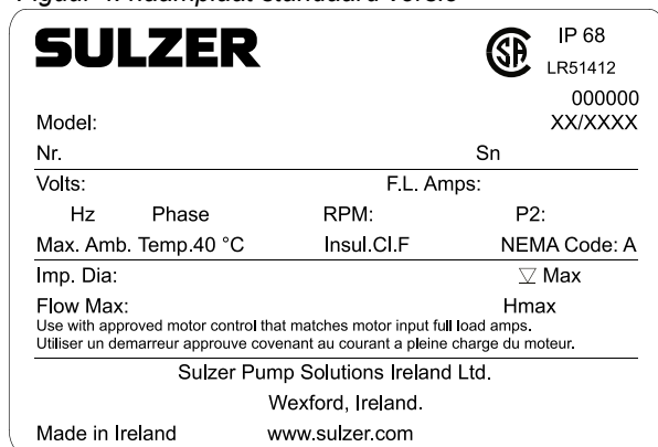
Figuur 4: naamplaat standaard versie
