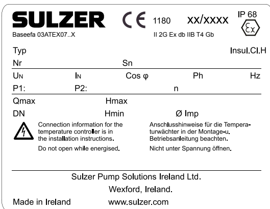
Figuur 1: naamplaat Ex-versie
