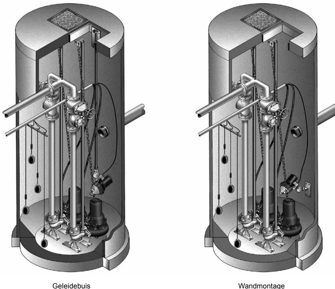
Geleidebuis
