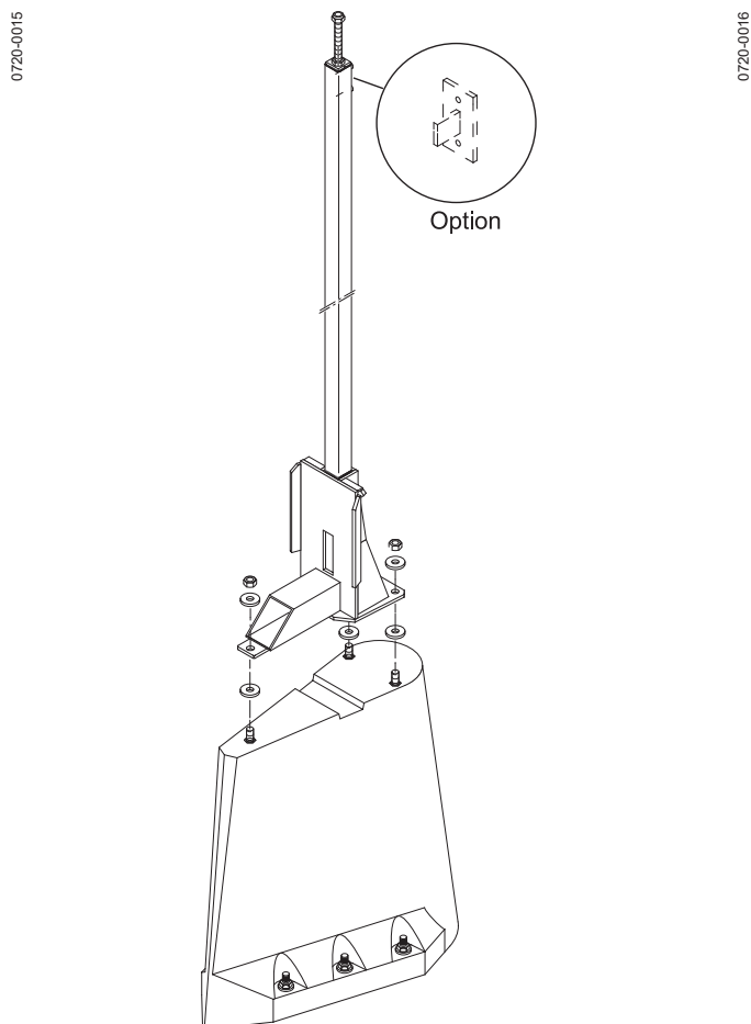
Εικόνα 14: Βίδωμα του συστήματος συνδέσμου
