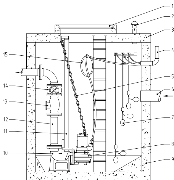
Rys. 3: Przykład instalacji, betonowy zbiornik ścieków
