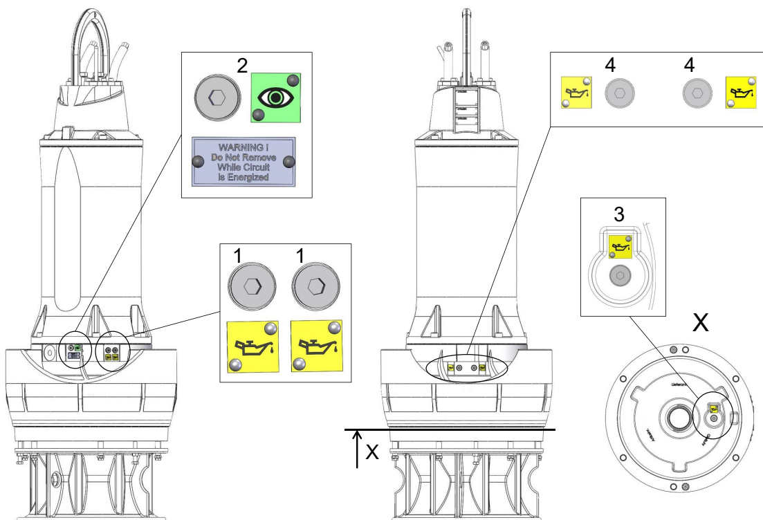
Obrázek 24. Plnění a vyprazdňování oleje AFLX / VUPX PE4
