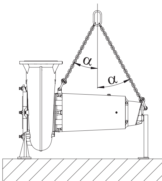
Obrázek 6. Horizontální přeprava
