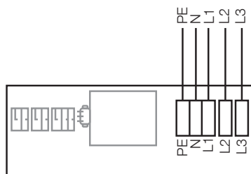
Fig 2. 3~ 400V
