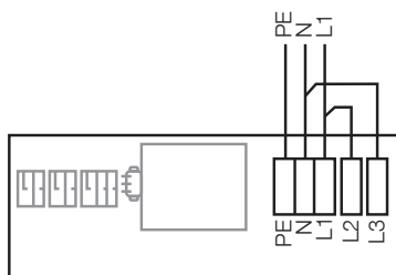
Fig 1. 1~ 230V
