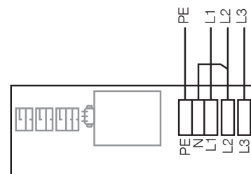
Fig 3. 3~ 230V
