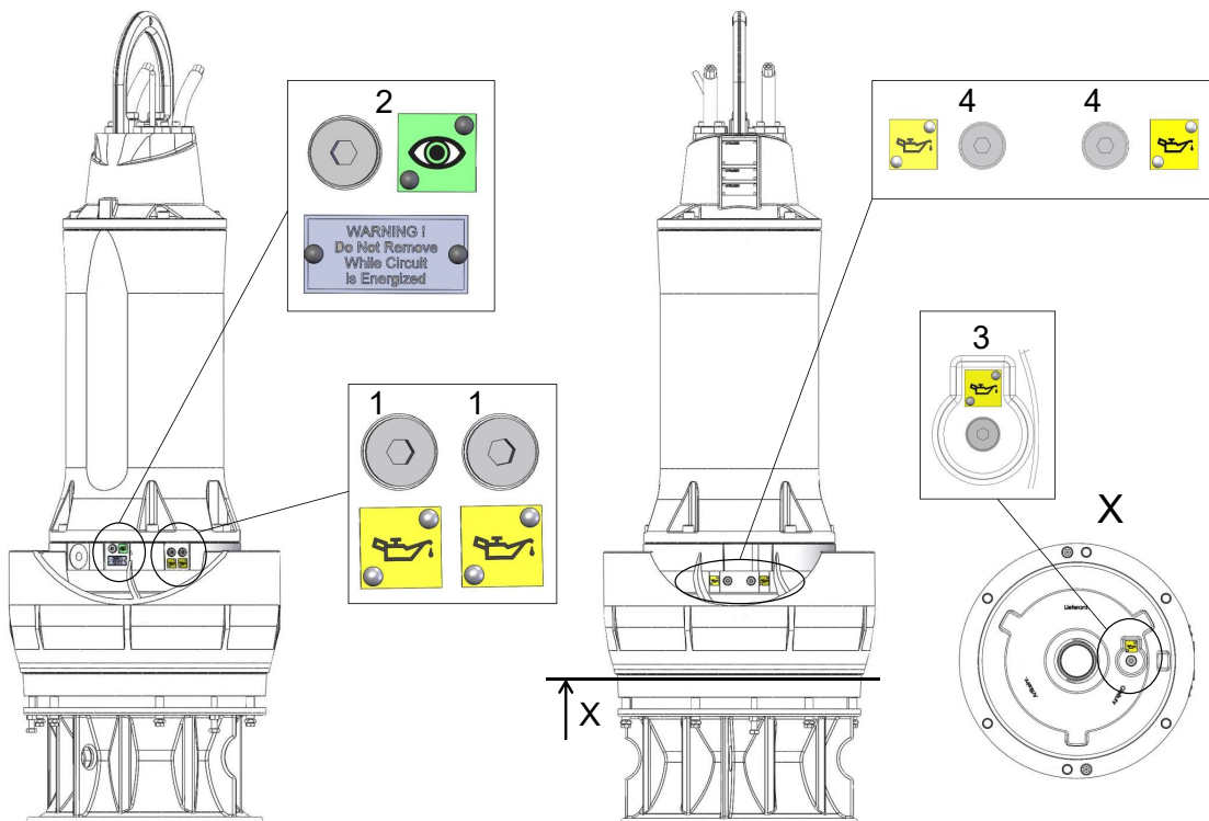
图 24. 润滑油的加注和排空 AFLX / VUPX PE4
