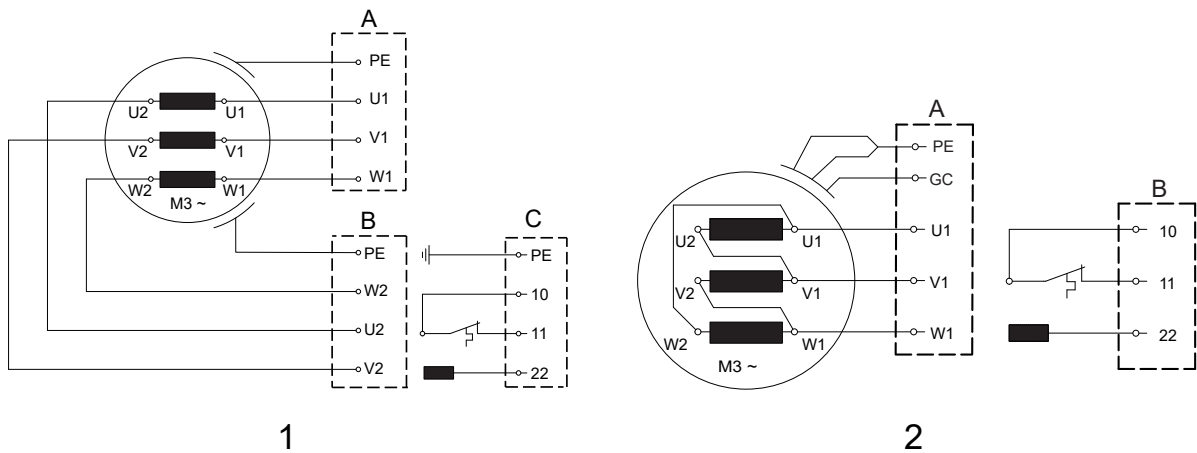
图 14.(1) 50 Hz：两根动力电缆和一根信号电缆。(2) 60 Hz：一根动力电缆和一根信号电缆。
