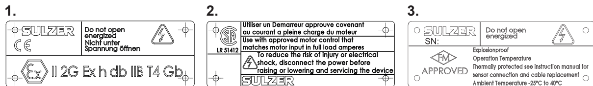
图 5.Ex 铭牌
